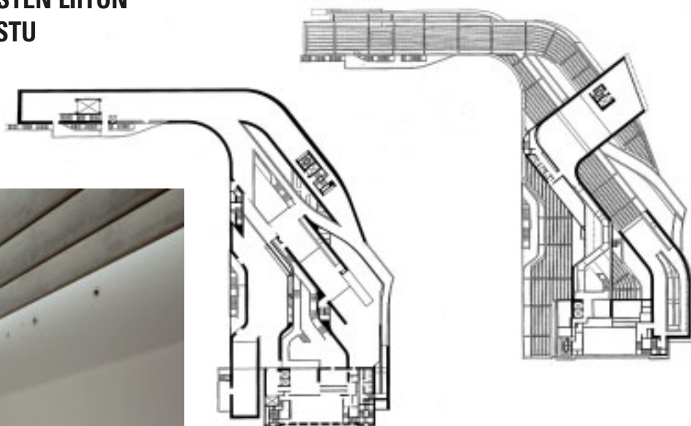
2 MAXXI, toisen ja kolmannen kerroksen pohjapiirrookset
