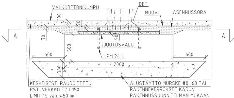
5 Rakennelleikkaus
