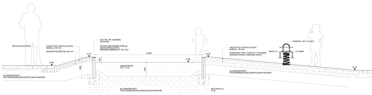
4 Hiekkalaatikko. Leikkauspiirros.
