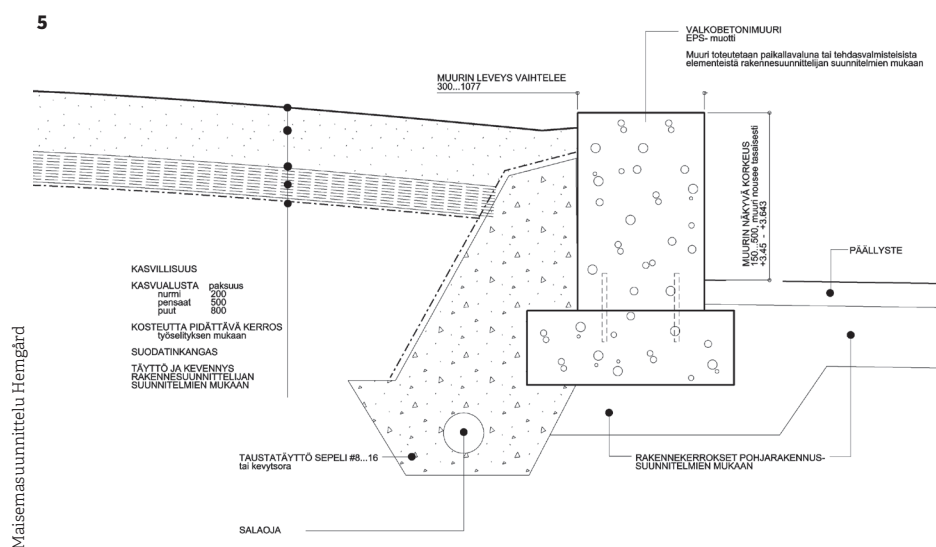
5 Betonimuuri. Leikkauspiirros.
