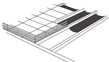
suojaverkko (verkkotyyppi T)
