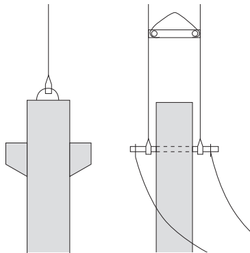
Pilarien nosto
