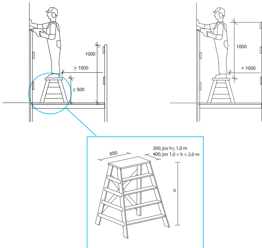
Kuva 11. Asennustyössä käytettävien työpukkien tulee olla tarkoitukseen soveltuvia ja hyväksyttyjä. Työpukkien käyttö esimerkiksi suojakaiteiden vieressä on vaarallista. Kun työpukkeja käytetään kaiteiden vieressä tulee kuvan mukaiset suojaetäisyydet täyttyä.
