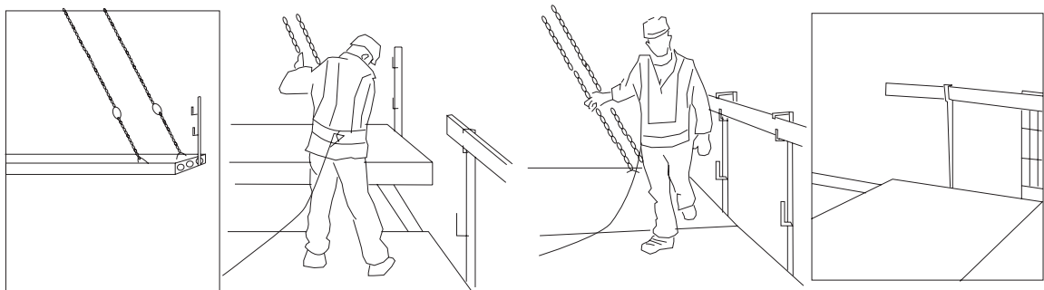
Kuva 18. Elementeissä olevat aukot suojataan välittömästi asennuksen jälkeen suojakaiteilla tai riittävän lujalla kannella. Laatastons asennuksen edetessä reunoille asennetaan kaiteet heti kun mahdollista.
