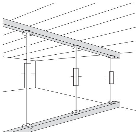
Kuori- ja liittolaatat tuetaan laataston alle asennettavien kannatinpalkkien ja säädettävien pystytukien avulla.
