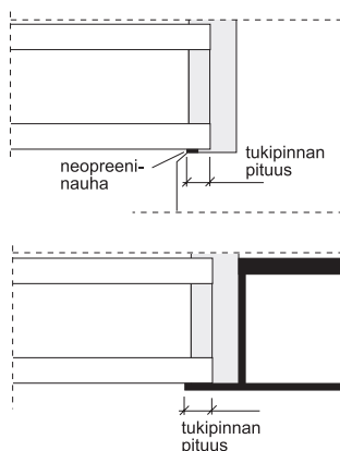
Laattojen tukipintoja.
