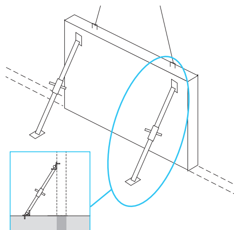
Seinäelementit tuetaan vähintään kahdella säädettävällä elementtituella.
