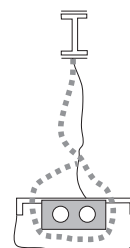
Kavennetut laatat, joissa ei ole nostolenkkejä, asennetaan myös liukukoukullisten nostoketjujen avulla. Nostosaksien turvaketju toimii varmistuksena.
