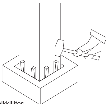
Holkkiiliitos.
