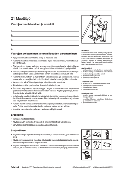
Kuva 2. Muottityön turvallisuusohje
