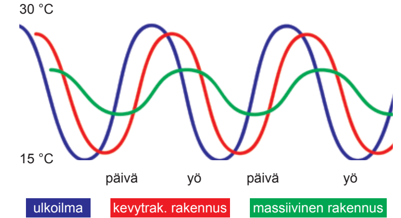
Massiivinen kivirakennus tasaa kesäajan sisälämpötilahuippuja 3-6 astetta ulkolämpötilaan nähden ja huippulämpötila viivästyy kuusi tuntia. Kevytrakenteisen rakennuksen tasaava vaikutus on pieni.
