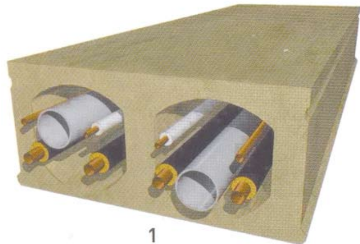
Ontelolaattojen onteloita voidaan käyttää IV-kanavina tai putkistojen asennukseen.
