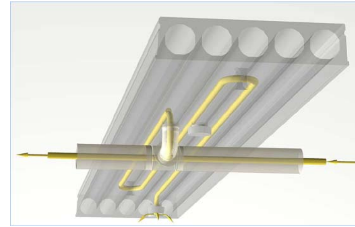
Kuva. Ontelolaitteen käyttäminen lämpövarastona TermoDeck-järjestelmässä.
