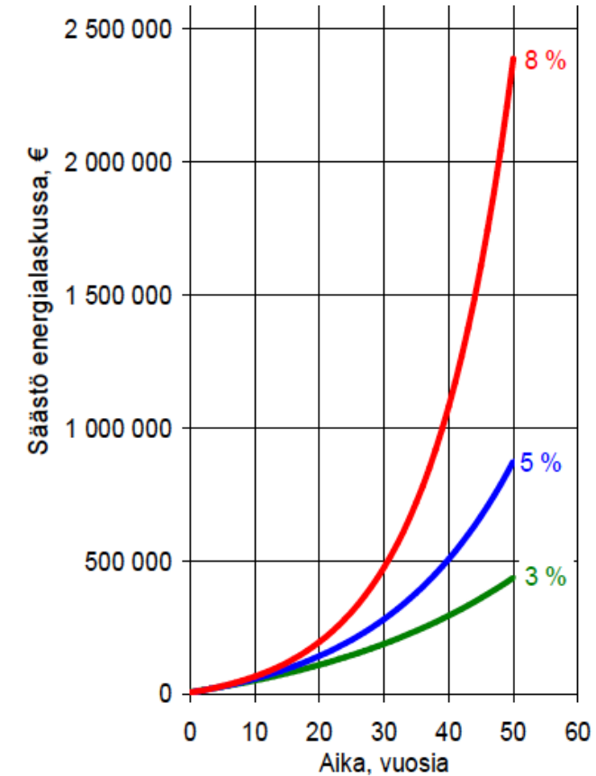
Kuva. Rakennusliike Reponen MERA- matalaenergiakerrostalon kumulatiivinen elinkaarikustannusero verrattuna Normikerrostalo 2005:een, kun energian reaalihintaa nousee 3%, 5% tai 8 % vuodessa.
