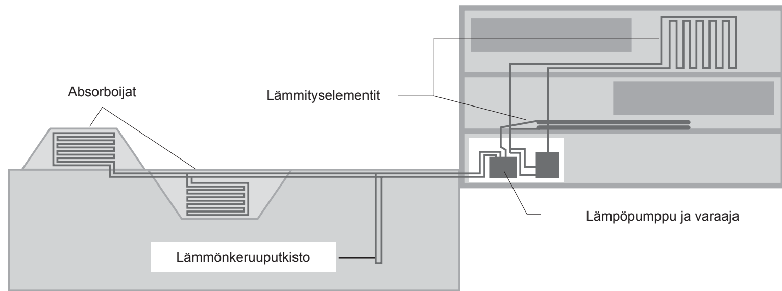
Maan päällä energiavarastoina voivat toimia esimerkiksi meluvallit ja näkösuojaseinät sekä betoniset tasakatot.
