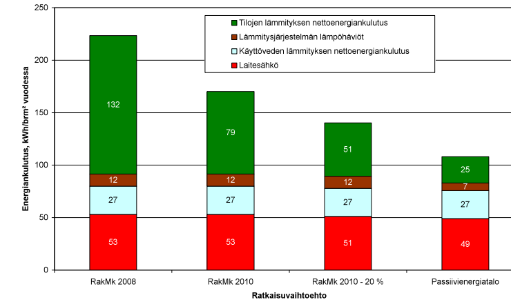
Harkkopientalon eri ratkaisuvaihtoehtojen vuotuiset ominaisenergiankulutukset.
