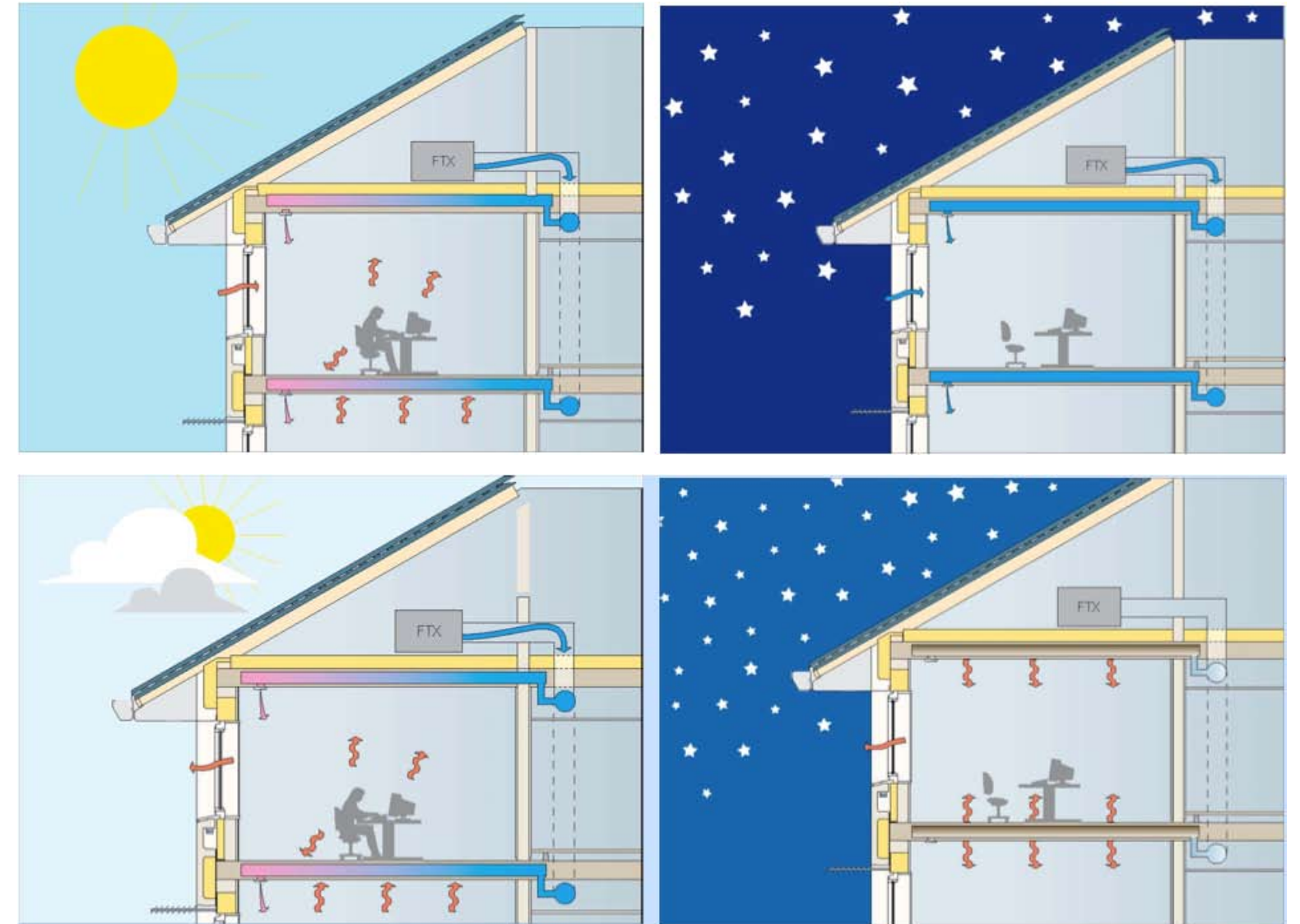
Massiivisten rakenteiden hyväksikäyttö rakennuksen lämpötilan tasaamisessa. TermoDeck-järjestelmän toiminta kesällä (ylempi kuva) ja talvella (alempi kuva).
