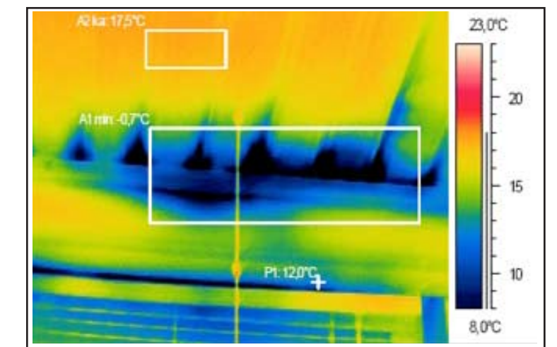
Lämpökamerakuva paljastaa seinän ja yläpohjan välisen lämpövuodon.
