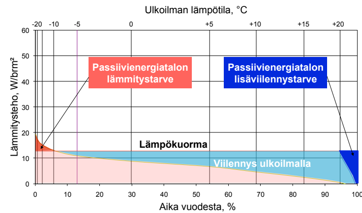
Kuva. Passiivenergiatalon lämmitys- ja viilennystarve.
