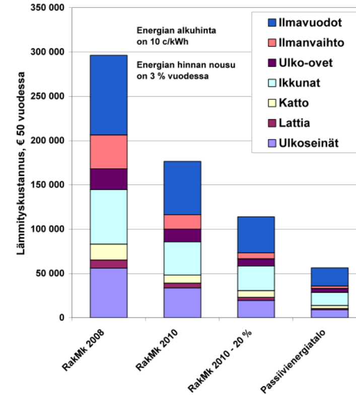
Kuva. Harkkopientalon lämmitysenergian kustannus 50 vuoden aikana, kun lämmitysenergian hinta on aluksi 10 c/kWh. Passiivenergiatalon lämmityskustannus on 120 000 € pienempi kuin vuoden 2010 alussa voimaan tulleiden rakennusten energiamääräysten mukaan rakennetun talon. Jos energiakustannus on jakson alussa 5 c/kWh, eroa syntyy tarkastelujaksolla passiivitalon hyväksi yhä 60 000 €.
