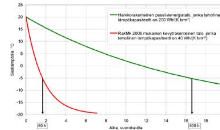
Hyvä lämmöneristys ja massiiviset sisä rakenteet bidastavat talon viilenemistä lämpökatkon aikana. Ulkoilman lämpötila on -20 astetta. /18/
